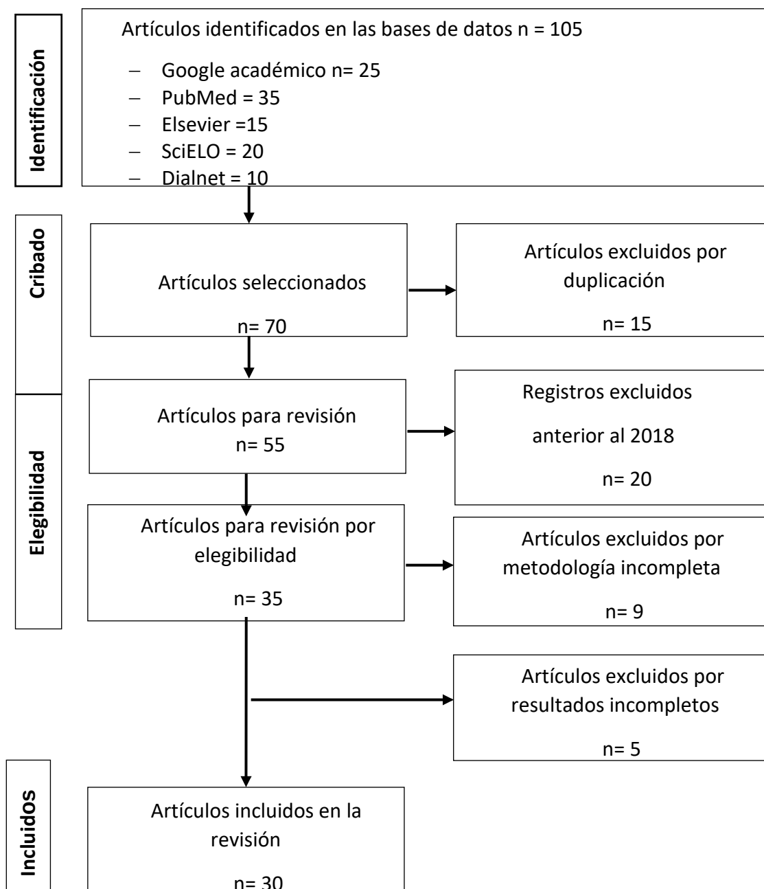
Gráfico 1. Diagrama PRISMA
